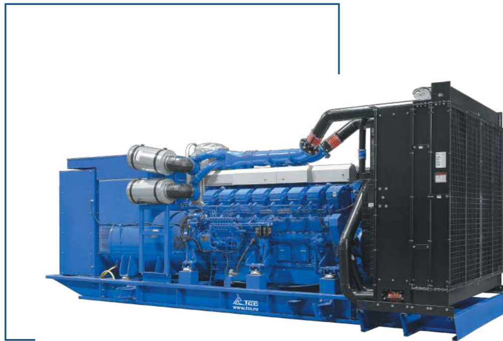
Дизельный генератор TMs 2200MC
